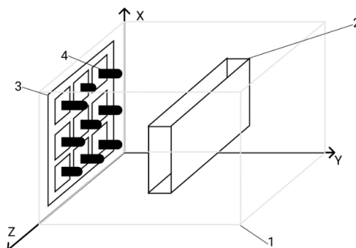
Рис 2. Ванна с каркасным фигурным анодом, состоящим из спиц - анодов
