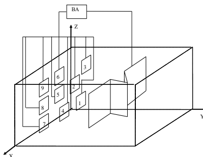
Рис 1. Многоанодная гальваническая ванна
