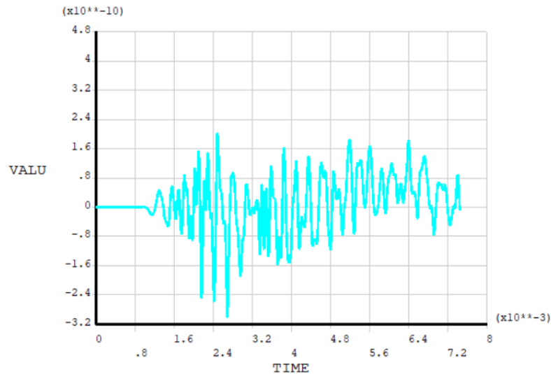
Рис.3. График перемещения VALU в точке 1 конструкции (м) во времени TIME (с)
