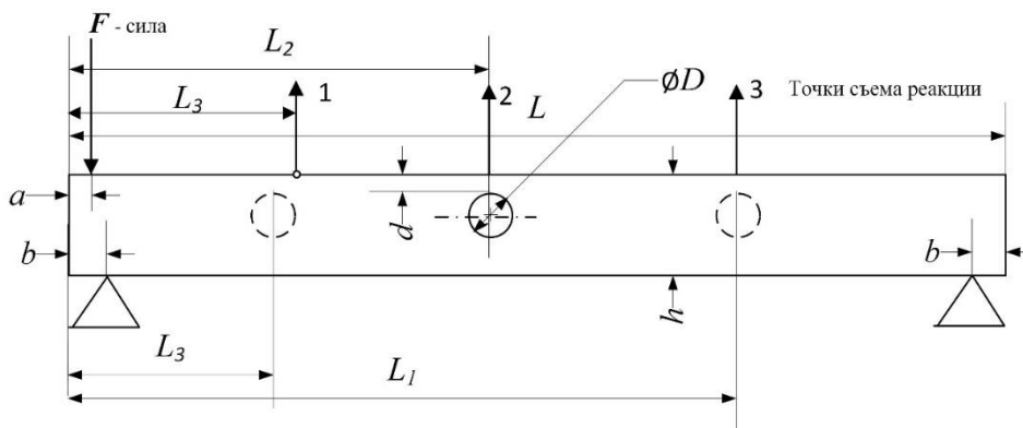
Рис.1. Моделируемая балочная конструкция
